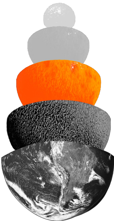
unterer Erdmantel
