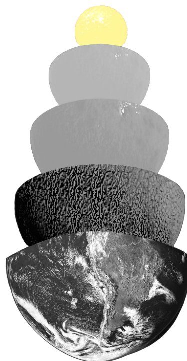
innerer Erdkern
