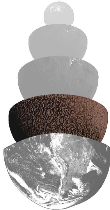
oberer Erdmantel
