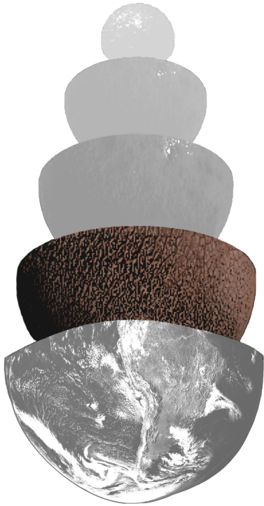
oberer Erdmantel
