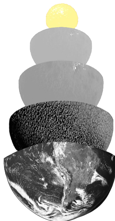
noyau interne
