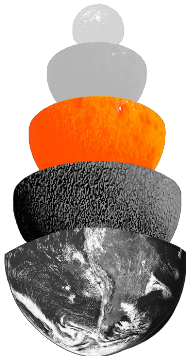
manteau inférieur
