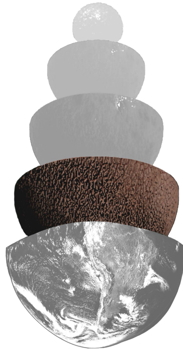
manteau supérieur
