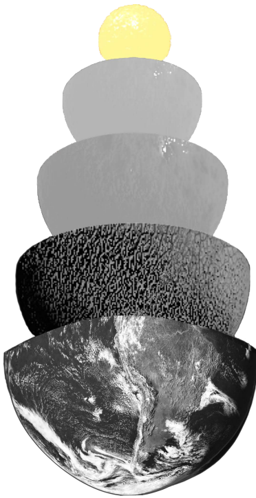
núcleo interno
