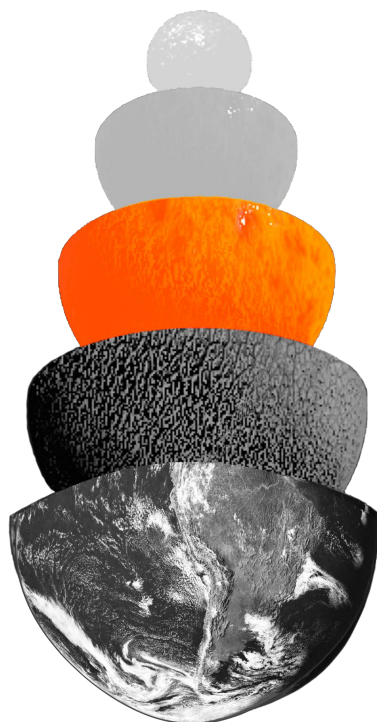
manto inferior
