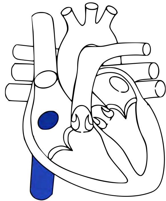
inferior vena cava
