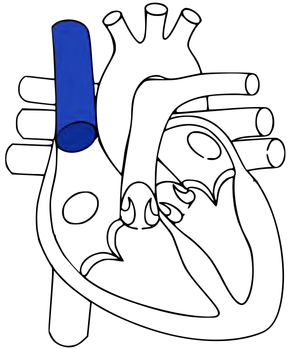
superior vena cava
